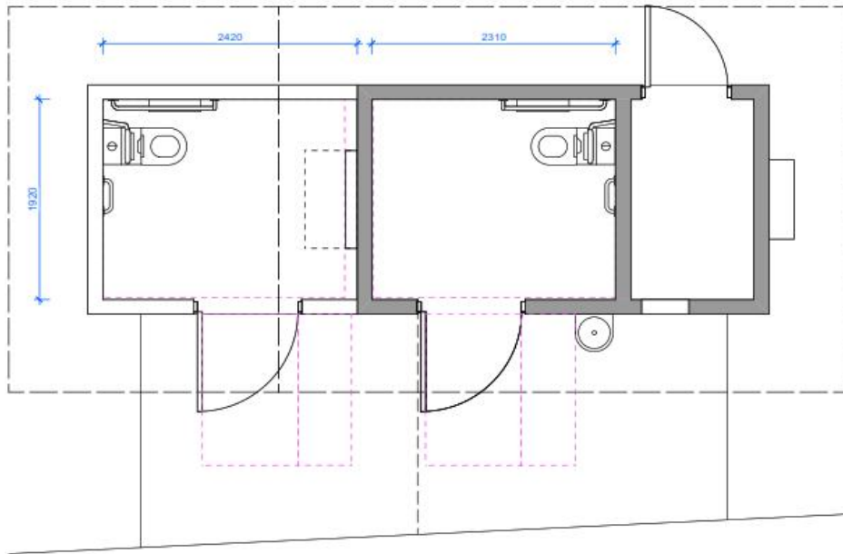
PLAN | 1 Scale: 1:50
